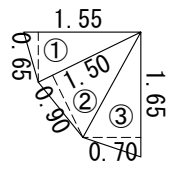
詳細図2-A
