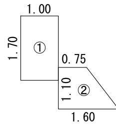
詳細図3-A
