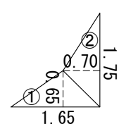
詳細図1-E
