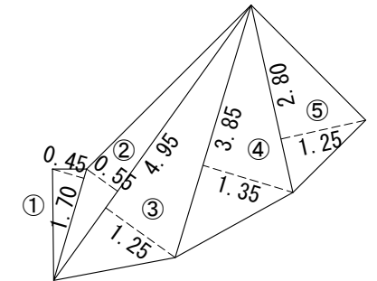
詳細図2-H
