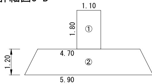
詳細図3-B
